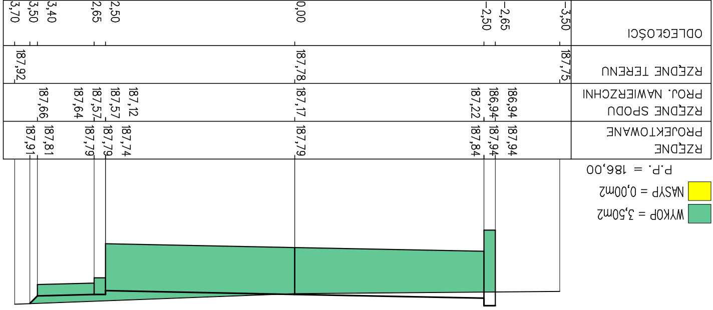
PK. 62,00 Skale 1:50/1:50
